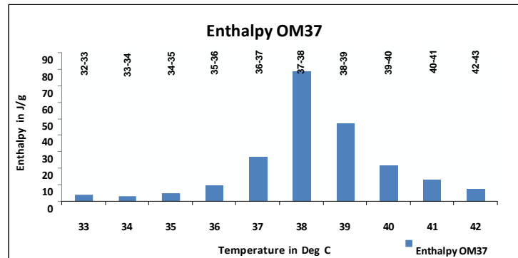
Enthalpy Vs Temp savE ® OM 37
