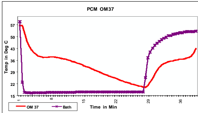
T-History graph savE ® OM 37
