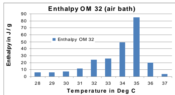
Enthalpy Vs Temp savE ® OM 32
