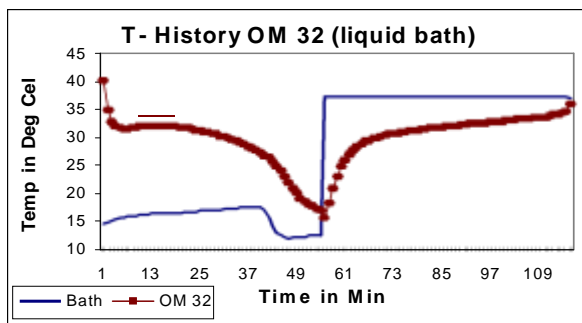
T-History graph savE ® OM 32
