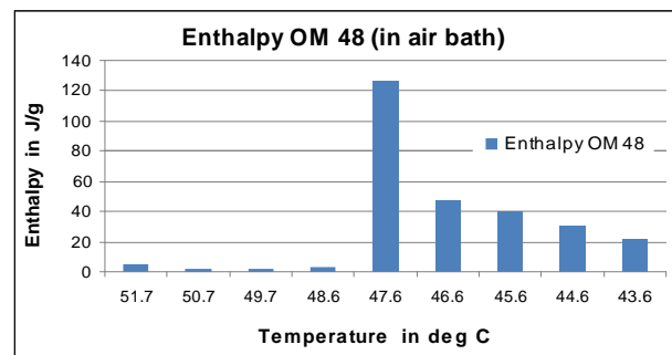
Enthalpy Vs Temp savE ® OM 48
