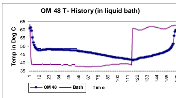
T-History graph savE ® OM 48
